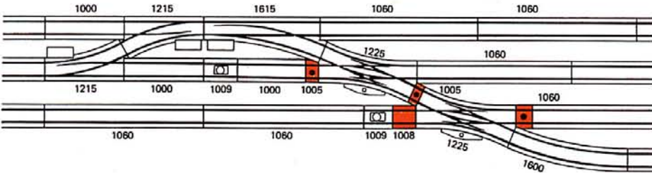
Bild 4-6 In Bahnhofsanlagen fügen sich DKW lückenlos ein, wenn die Weichen 1605 oder 1615 ohne Einpassgleise also direkt an eine DKW angeschlossen werden. Weiterbau mit 30° Weichen oder Kreuzungen kann in gewohnter Weise erfolgen.
