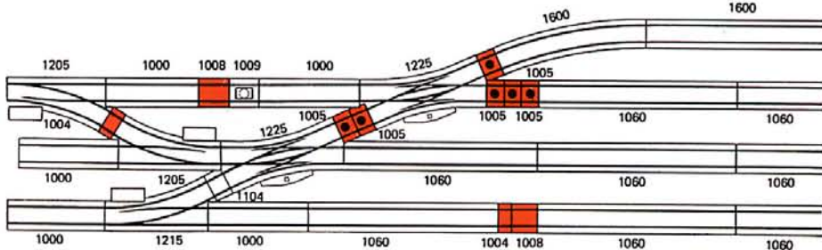
Bild 2 Weichenstrasse Kombination DKW - 30° Weiche, Ausgleich mit Bogengleis 1104, 7,5°, Gleisabstand 185.
