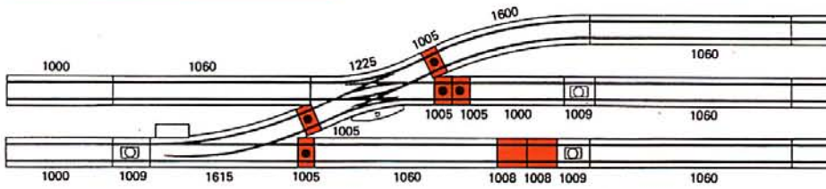
Bild 1 Eine DKW mit Anschluss an Weiche 1615
